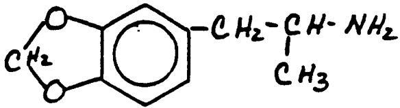
MDA
